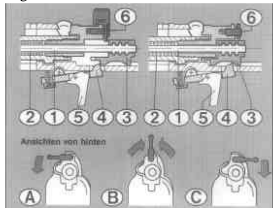
Sicherung bei Mauser 98
